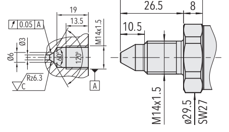
8292.XX.XX29.XX.XX.XX (> 600 bar)
