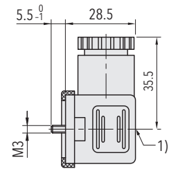
8292.XX.XXXX.XX.XX.58
