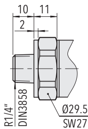
8292.XX.XX19.XX.XX.XX (≤ 600 bar)
